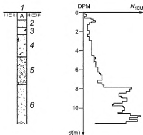
1 — наполнение, 2 — глинистый песок, гравий, сусесь; 3 — торф; 4 — озерный мергель с остатками растений; 5 — глинистый озерный мергель; 6 — супесчаный крупный песок с мелким гравием; d — глубина
