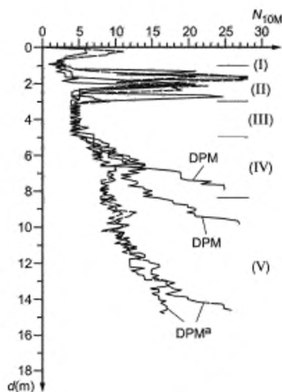
DPM — динамическое зондирование без бурового раствора; DPM^B — динамическое зондирование с буровым раствором; I — почва; II — гравий; III — переработанная выветренная глина; IV — выветренная глина; V — неветренная глина; d — глубина
