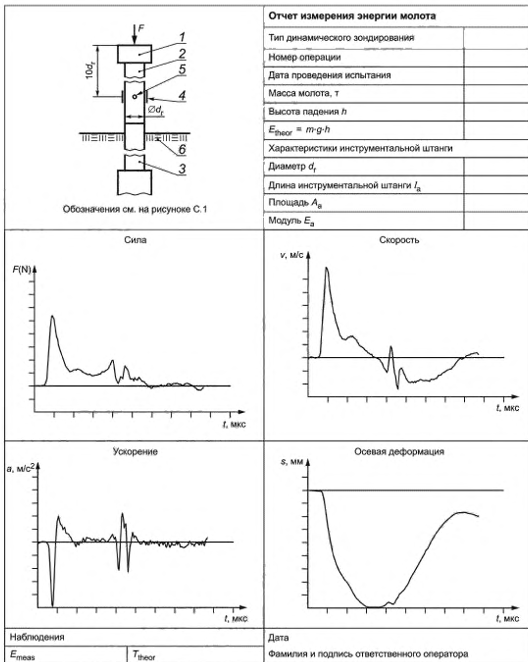
Рисунок С.2 — Пример отчета измерения энергии молота
