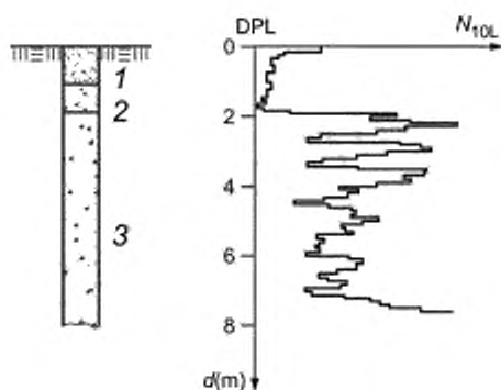
1 — супесь, песчаная, 2 — супесь; 3 — гравий; d — глубина
