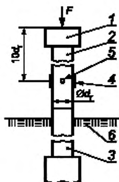
1 — наковальня; 2 — специально оборудованный участок штанг (измерительная штанга); 3 — забивные штанги, 4 — тензометр (измерительный преобразователь); 5 — акселерометр; 6 — грунт; F — сила, d_s — диаметр штанги
