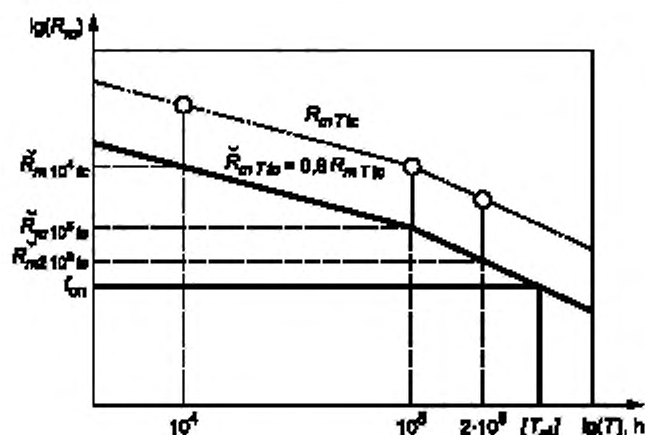
Рисунок А.1 — Диаграмма для определения [T_{adj}]
