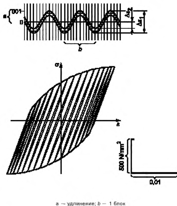
Рисунок В.1 — Характеристика соотношения напряжений и деформации по Доулингу [2]
