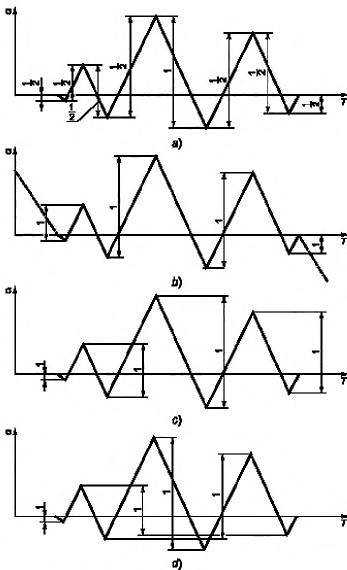
Рисунок В.5 — Варианты оценки величин в ОГП
