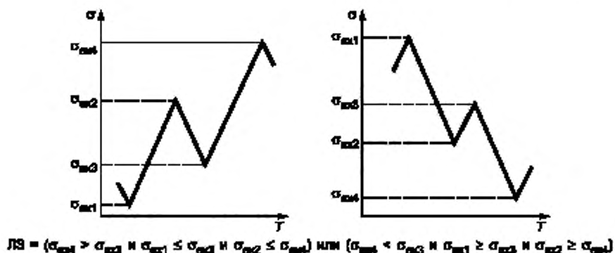
Рисунок В.3 — Критерий для цикла нагружения с диапазоном \Delta\sigma_{ex} = |\sigma_{ex2} - \sigma_{ex3}| с применением метода дождевого потока и метода парной амплитуды
