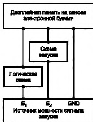
Рисунок 1 — Блок-схема для разъяснения напряжения питания
