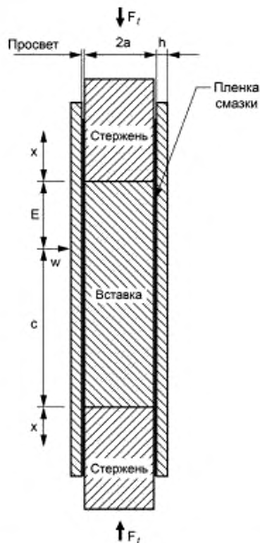
Рисунок 2 — Схематическое изображение вставки с одноосевой нагрузкой [см. 1]
