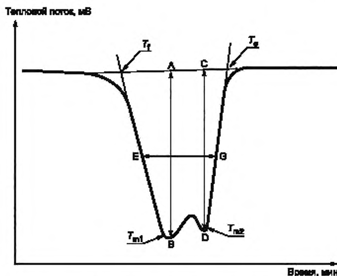
Рисунок 1 — ДСК-кривая нагревания
