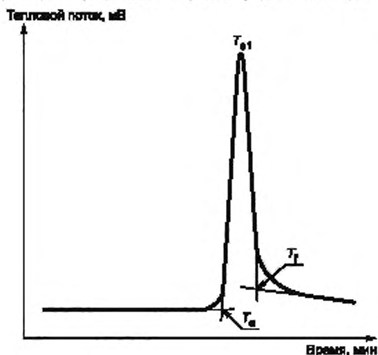
Рисунок 2 — ДСК-кривая охлаждения
