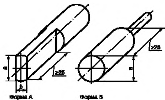
Рисунок 5 — Щупы (см. 9.2.4.5)
