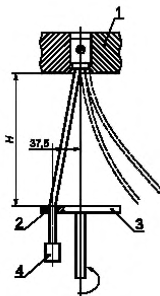
Рисунок 4 — Установка для испытания проводников на изгиб (см. 9.2.4.3.)
