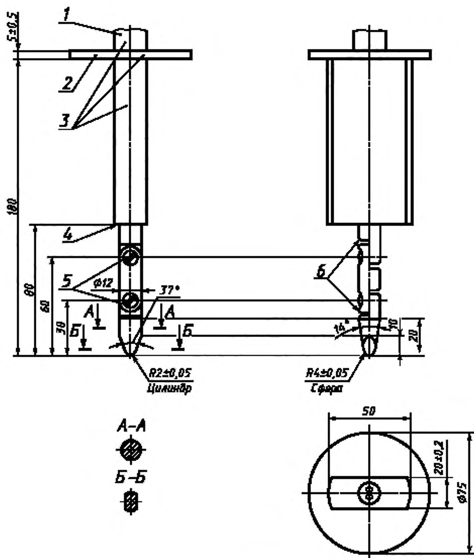
1 – рукоятка; 2 – упор; 3 – изолирующий материал; 4 – упорная поверхность; 5 – соединения; 6 – скруглить кромки
