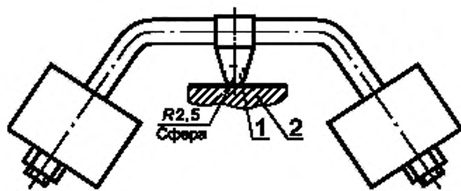
Рисунок 3 — Установка для испытаний давлением шарика (см. 9.2.1.3.1)
