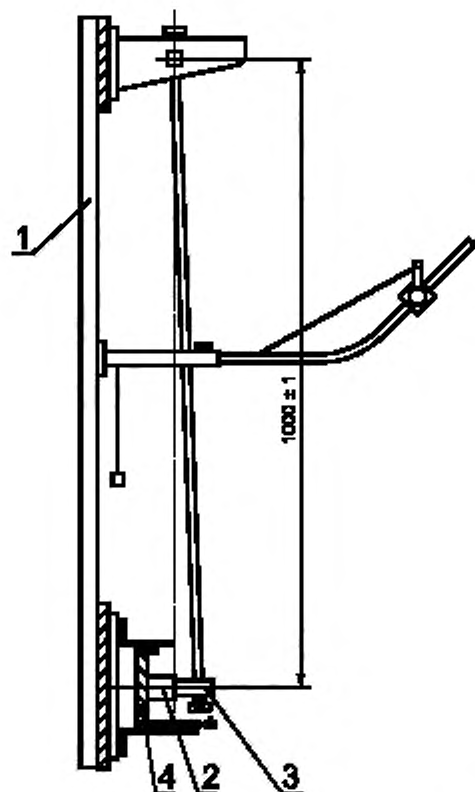
1 – опора; 2 – образец; 3 – ударный элемент; 4 – монтажная опора
