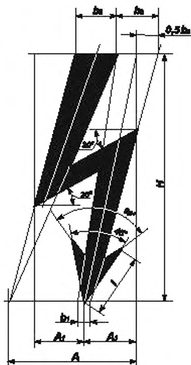
Рисунок Л.1 – Графический символ электрического напряжения
