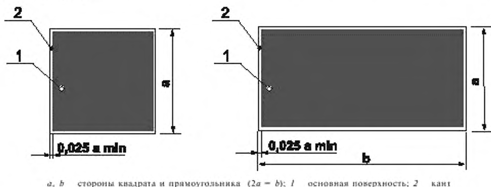
Рисунок 5 – Основа цветографического изображения и соотношение размеров эвакуационных знаков безопасности и знаков безопасности медицинского и санитарного назначения
