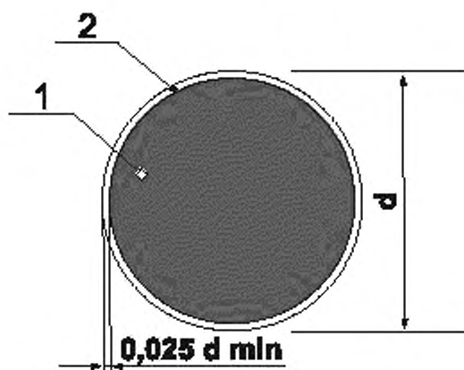
d диаметр круга; 1 основная поверхность; 2 кант
