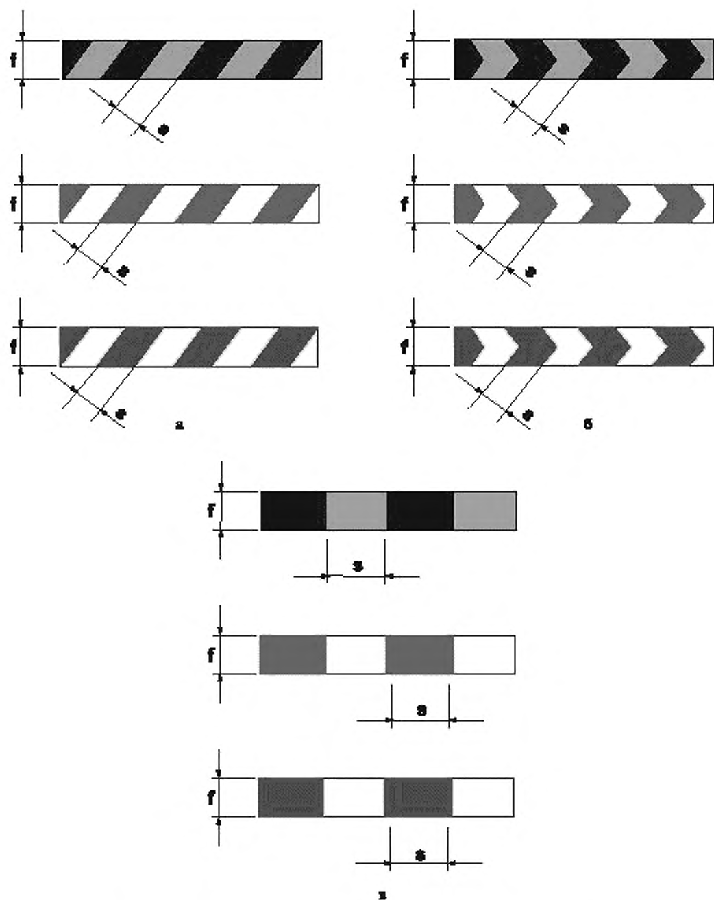
а - расположение полос наклонно, б - расположение полос зигзагообразно в виде «елочки», в - расположение полос прямо (вертикально или горизонтально), Г - поперечный размер сигнальной разметки, s - ширина полосы сигнального цвета.
