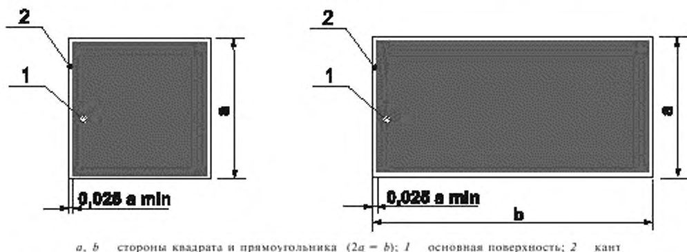
Рисунок 6 – Основа цветографического изображения и соотношение размеров указательных знаков безопасности
