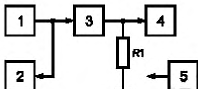
1 — генератор сигналов НЧ; 2 — милливольметр НЧ; 3 — возбудитель передатчика; 4 — милливольметр ВЧ; 5 — анализатор спектра ВЧ; R1 — резистор сопротивлением (75 \pm 4) Ом
