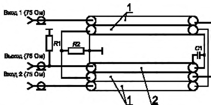
Рисунок Г.2 — Электрическая схема сумматора противофазных сигналов
