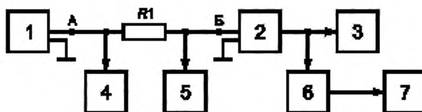
1 — генератор сигналов НЧ; 2 — передатчик; 3 — эквивалент антенны; 4, 5 — милливольтметры НЧ; 6 — элемент связи; 7 — модулометр; R1 — резистор сопротивлением (600±3) Ом
