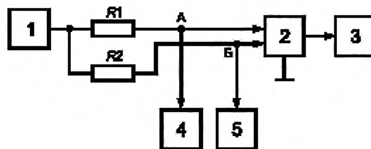
1 — генератор сигналов НЧ; 2 — передатчик; 3 — эквивалент антенны; 4, 5 — милливольтметры НЧ; R1, R2 — резисторы сопротивлением (300±0,3) Ом
