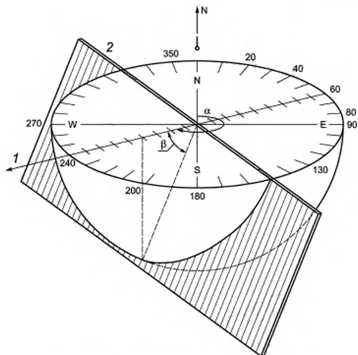
1 — линия падения; 2 — линия простирания (плоскости разрыва, пласта); \alpha — направление падения (азимут падения) = 240^\circ ; \beta — падение (угол падения) = 50^\circ вектор плоскости разрыва 240/50
