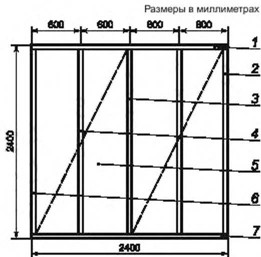
Рисунок 1 — Схема стеновой панели
