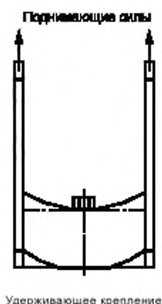
Рисунок 2 — Пояснение искривления нижнего опорного ребра
