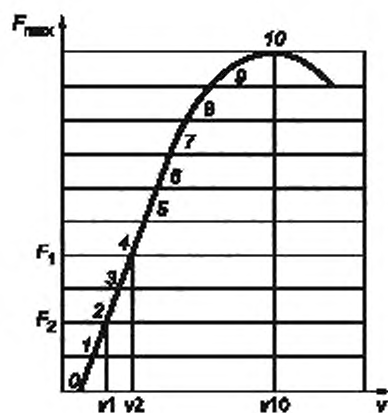
Рисунок 4 — Метод испытания
