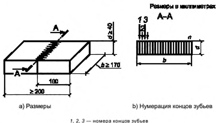
Рисунок А.1 — Испытуемые образцы для испытания на расслоение зубчатых соединений в слоях
