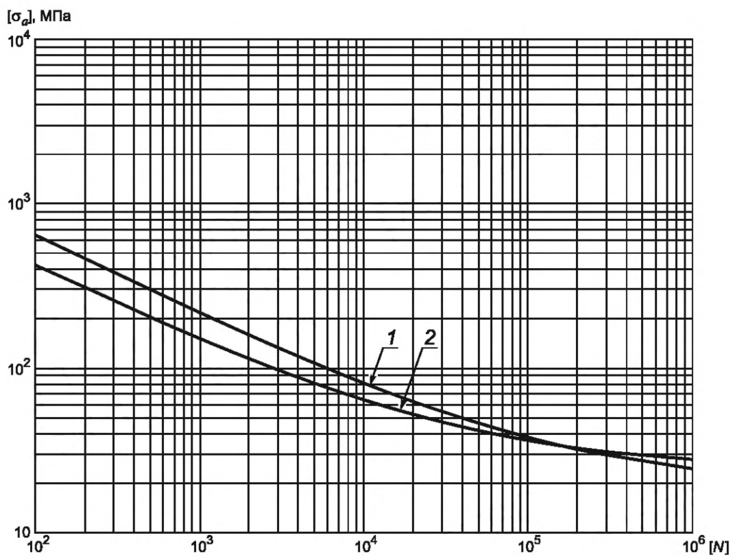
1 — ВТ1-0, ВТ1-00 при A = 0,46 \cdot 10^5 МПа, B = 45,2 МПа, T = 300 °С; 2 — ОТ4-0 при A = 0,33 \cdot 10^5 МПа, B = 58,8 МПа, T = 400 °С
