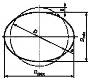
Рисунок А.3 — Общая некруглость
