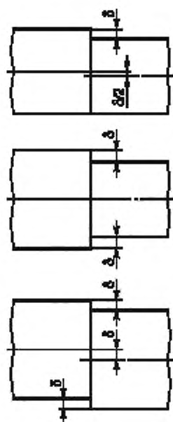
б — кольцевые сварные швы
