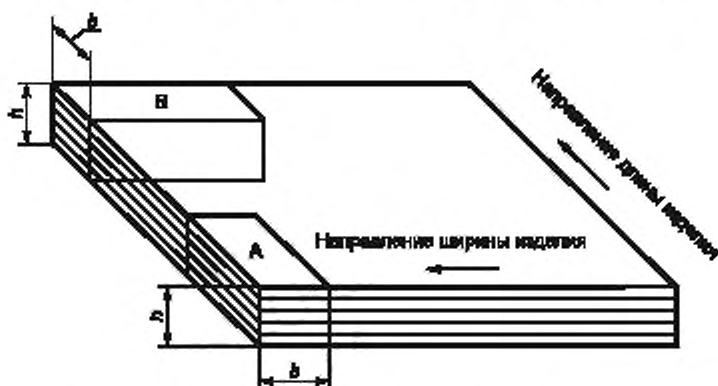
Рисунок ДА.4 — Схема формирования (вырезания) образцов
