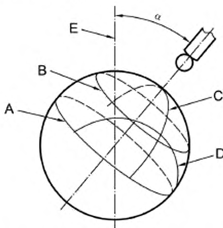
A — целевая плоскость сканирования 1; B — целевая плоскость сканирования 2; C — целевая плоскость сканирования 3; D — целевая плоскость сканирования 4; E — ось пинноли
