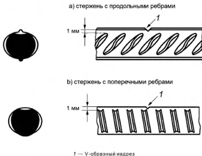
Рисунок А.1 — Надрез на арматурном стержне
