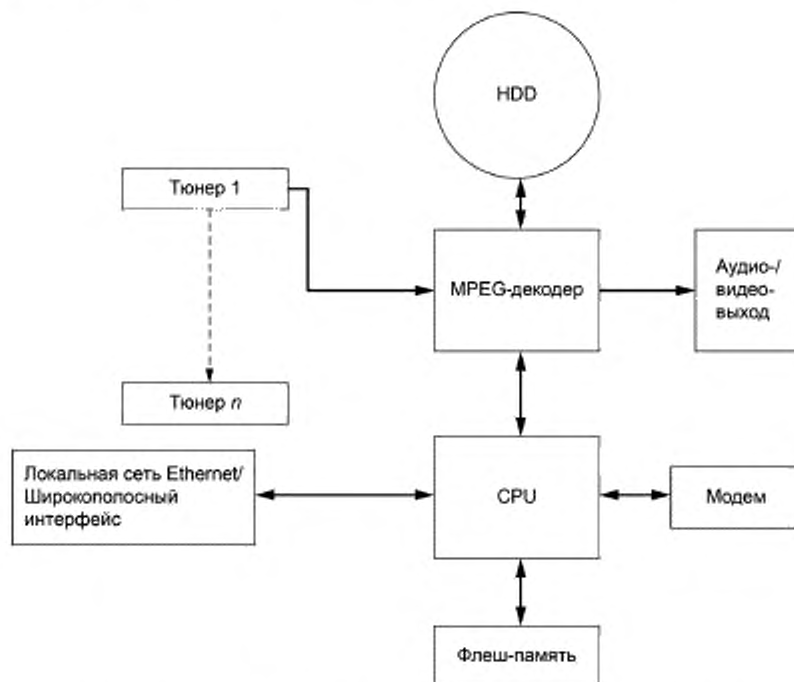
Рисунок А.1 — Блок-схема общих функциональных частей STB
