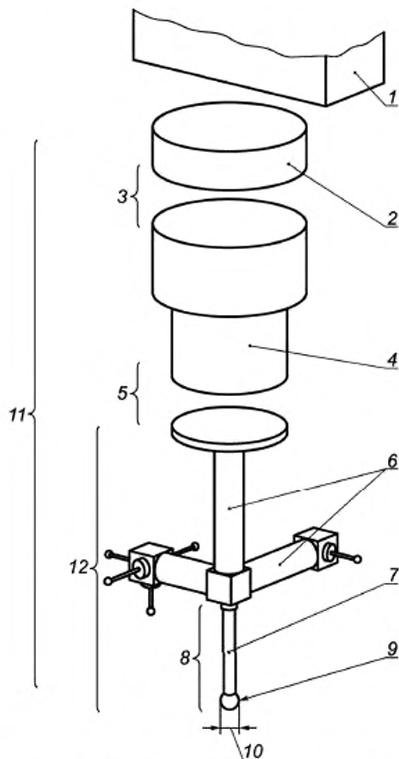
Рисунок 1 — Зондирующая система
