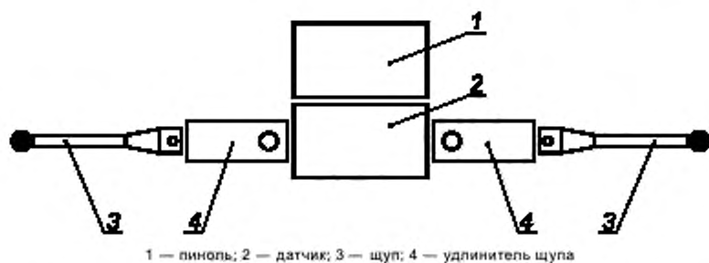
Рисунок 7 — Многощуповая зондирующая система (два одиночных щупа)
