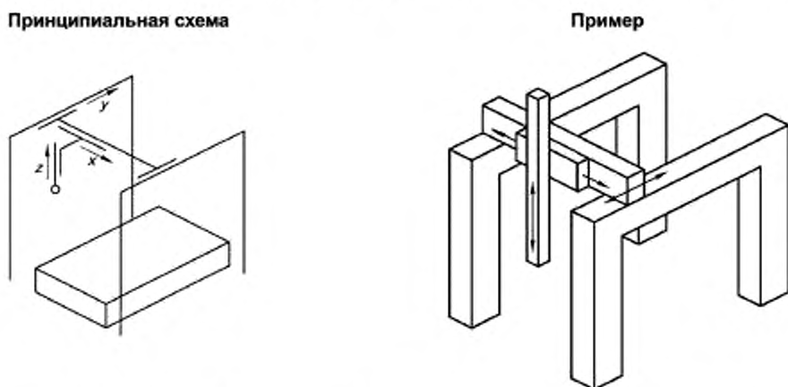
Рисунок А.3 — Портальная КИМ
