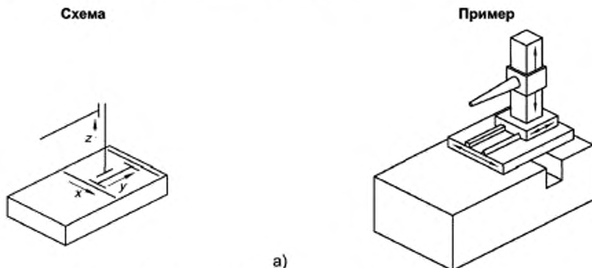
Рисунок A.9, лист 1 — КИМ с горизонтальной рукой и неподвижным столом
