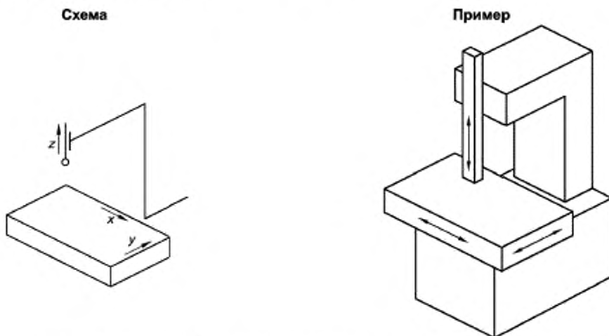
Рисунок А.7 — КИМ стоечного типа
