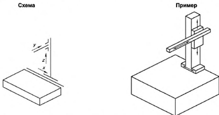
Рисунок A.8 — КИМ с горизонтальной пинолью
