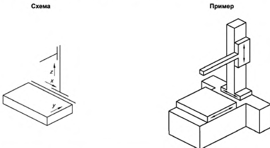
Рисунок А.10 — КИМ с горизонтальной рукой и подвижным столом
