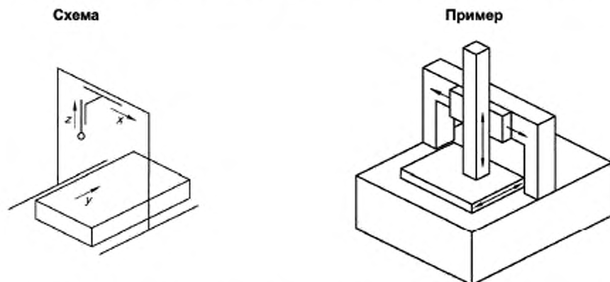
Рисунок А.5 — КИМ с неподвижным мостом
