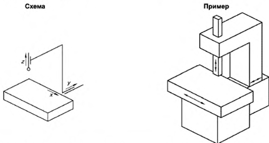
Рисунок А.6 — Консольная КИМ с подвижным столом
