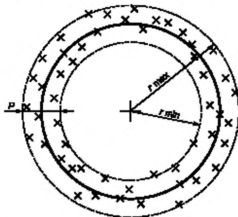
Рисунок 15 — Погрешность зондирования
