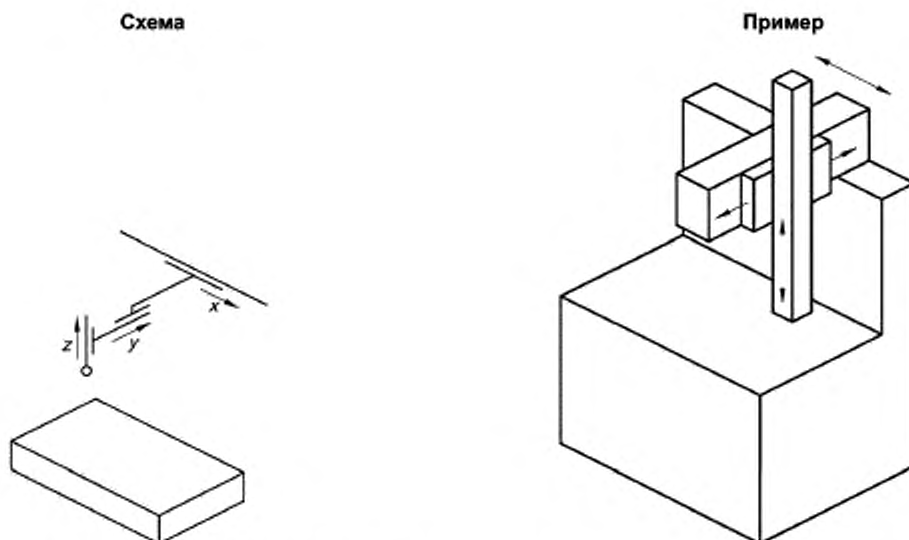
Рисунок А.1 — Консольная КИМ с неподвижным столом
