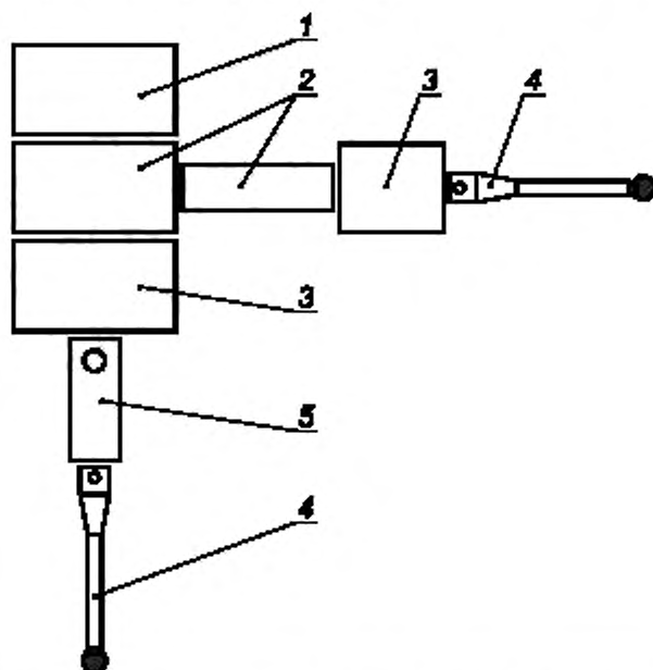
1 — линоль; 2 — удлинитель датчика; 3 — датчик; 4 — щуп; 5 — удлинитель щупа
