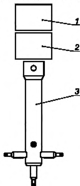
1 — пиноль; 2 — датчик; 3 — щуп в форме звезды
