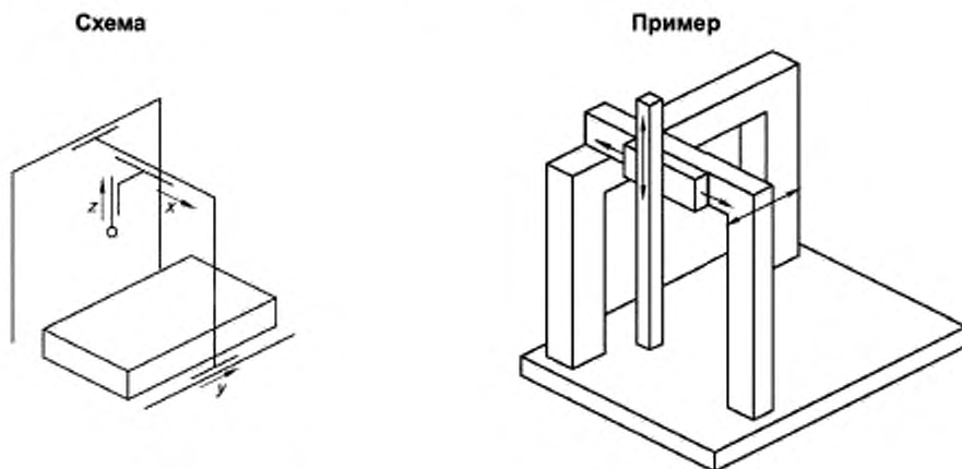
Рисунок А.4 — КИМ с L-образным мостом
