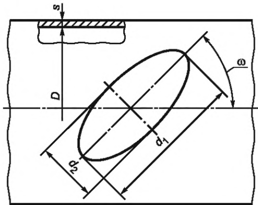
Рисунок А.16 — Отверстие для овального штуцера, перпендикулярного поверхности обечайки
