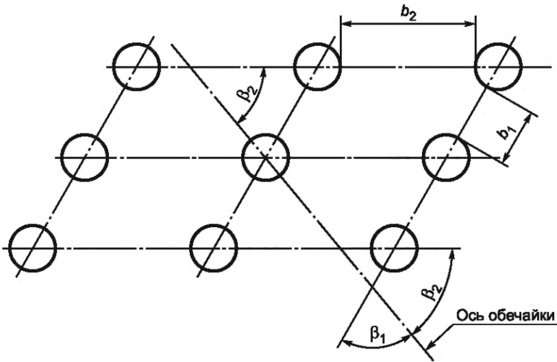
Рисунок А.17 — Ряды отверстий
