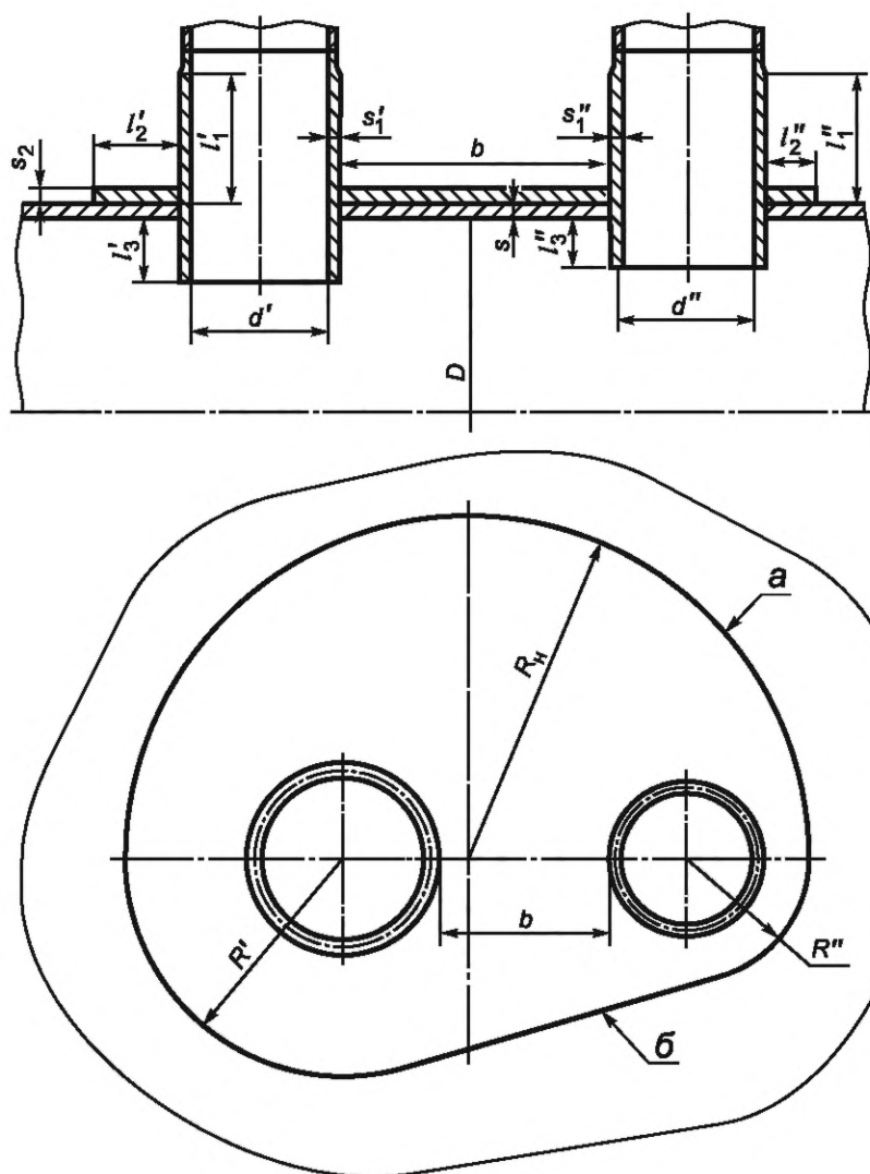
Рисунок А.9 — Совместное укрепление взаимовлияющих отверстий
