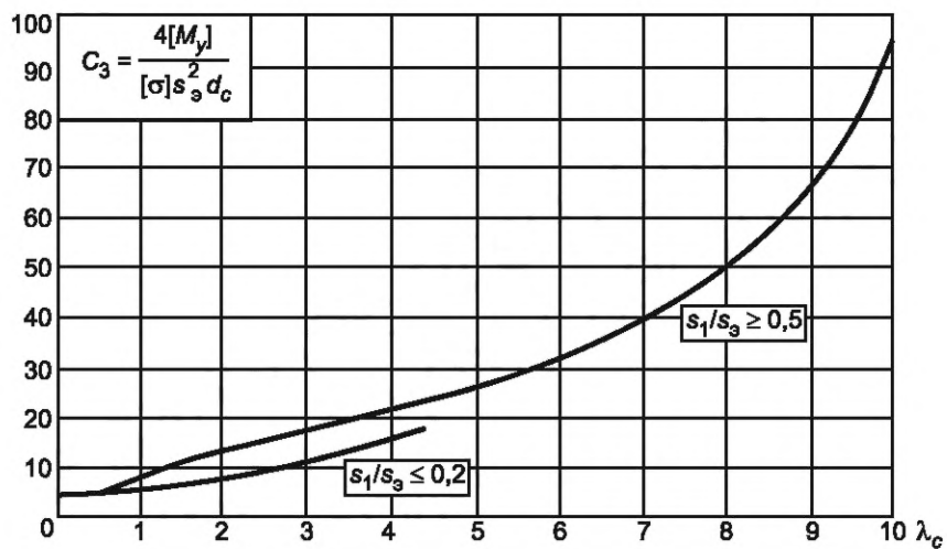
Рисунок Б.4 — График для определения C_3
