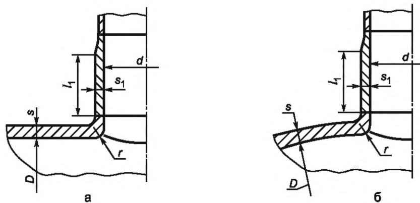
Рисунок А.6 — Укрепление отверстий отбортовкой
