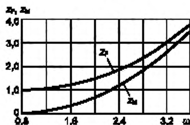
Рисунок 19 — Коэффициенты z_F и z_M
