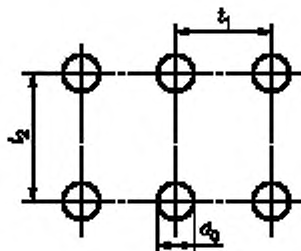
Рисунок Ж.1 — Расположение отверстий по вершинам прямоугольников
