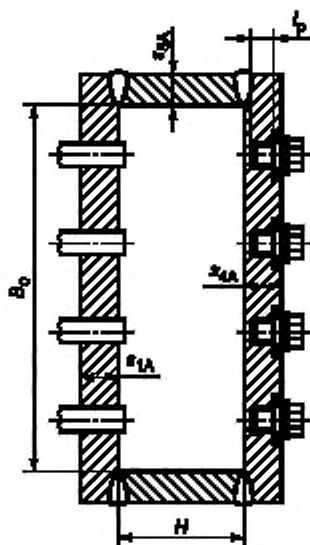
Рисунок 21 — Сварная камера без перегородок
