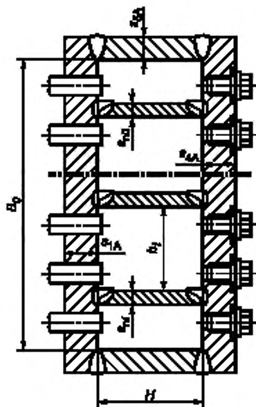
Рисунок 23 — Сварная камера с перегородками
