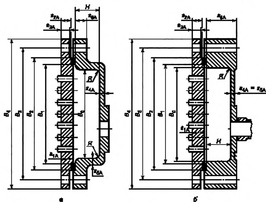
Рисунок 16 — Камера разъемной конструкции с литой крышкой
