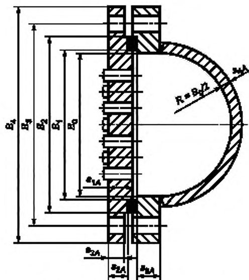
Рисунок 18 — Камера разъемной конструкции со сварной полцилиндрической крышкой
