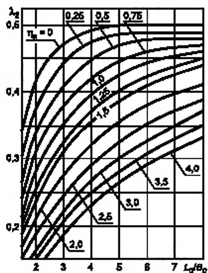
Рисунок И.2 — График коэффициента \lambda_2
