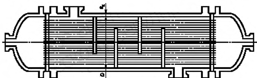
Рисунок 1 — Аппарат с неподвижными трубными решетками
