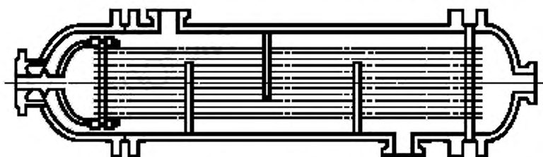
Рисунок 6 — Аппарат с компенсатором на плавающей головке
