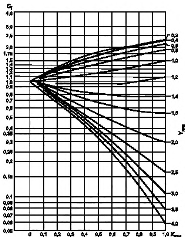
Рисунок А.1 — Параметр жесткости компенсатора C_T
