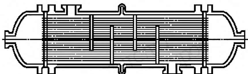
Рисунок 2 — Аппарат с компенсатором на кожухе
