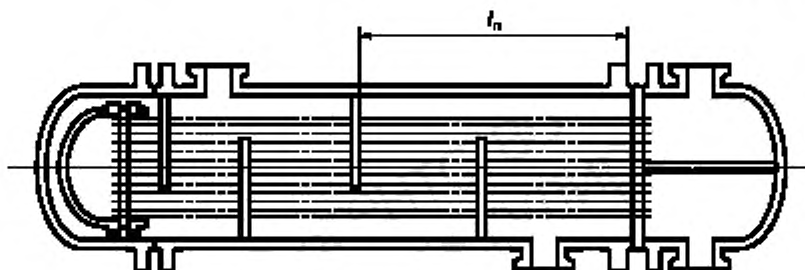
Рисунок 5 — Аппарат с плавающей головкой
