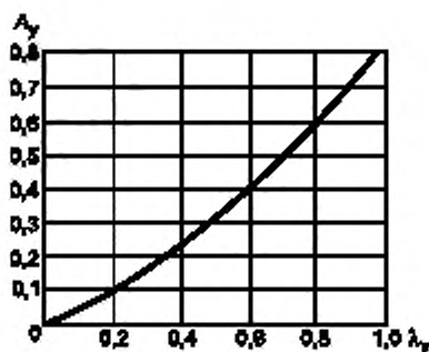
Рисунок 12 — Коэффициент для определения максимального прогиба трубы
