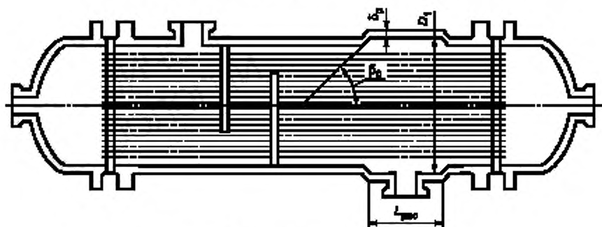
Рисунок 3 — Аппарат с расширителем на кожухе
