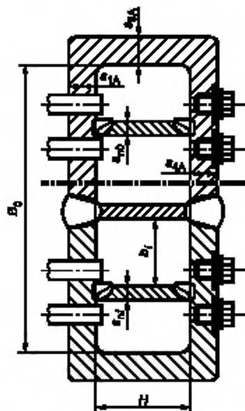
Рисунок 24 — Штампованная камера с перегородками
