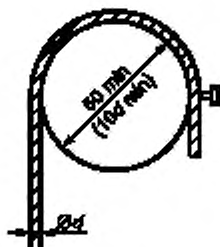
Рисунок 1 — Устройство для удерживания испытуемого образца корда
