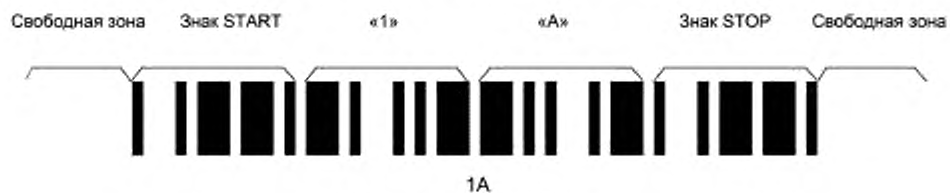
Рисунок 1 — Символ Code 39
