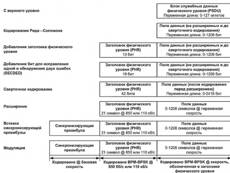
Рисунок 4 — Процесс кодирования блока PPDU
