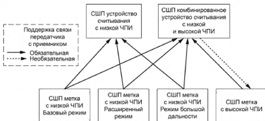
Рисунок A.3 — Взаимодействие физических уровней сверхширокополосного радиointерфейса с низкой и высокой ЧПИ
