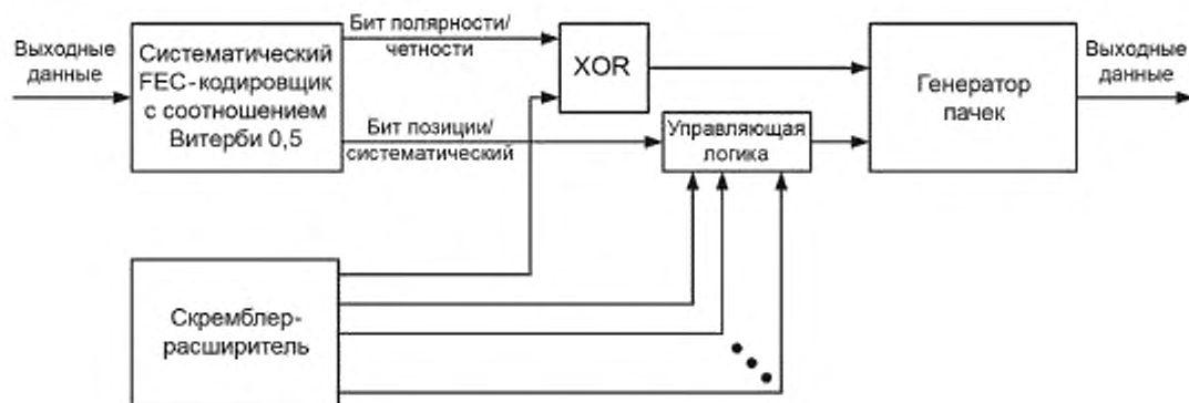
Рисунок 10 — Опорный модулятор символов**
