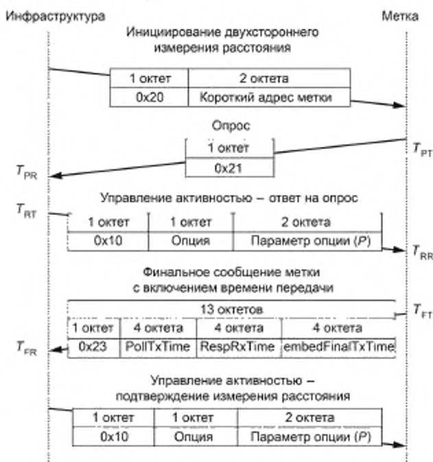
Рисунок 28 — Двухстороннее измерение расстояния
