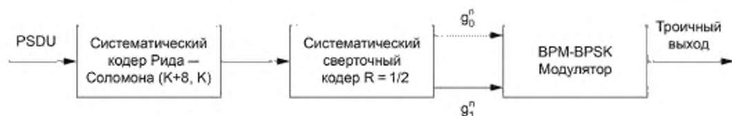
Рисунок 9 — Процесс кодирования поля данных
