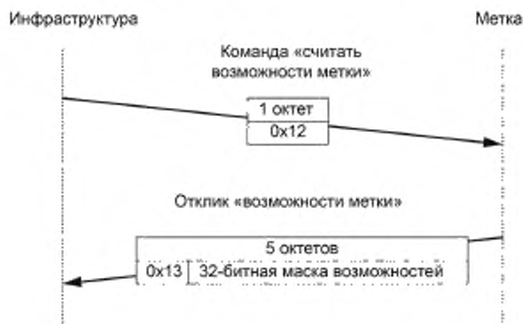
Рисунок 24 — Команда «считать возможности метки» (read tag capabilities)
