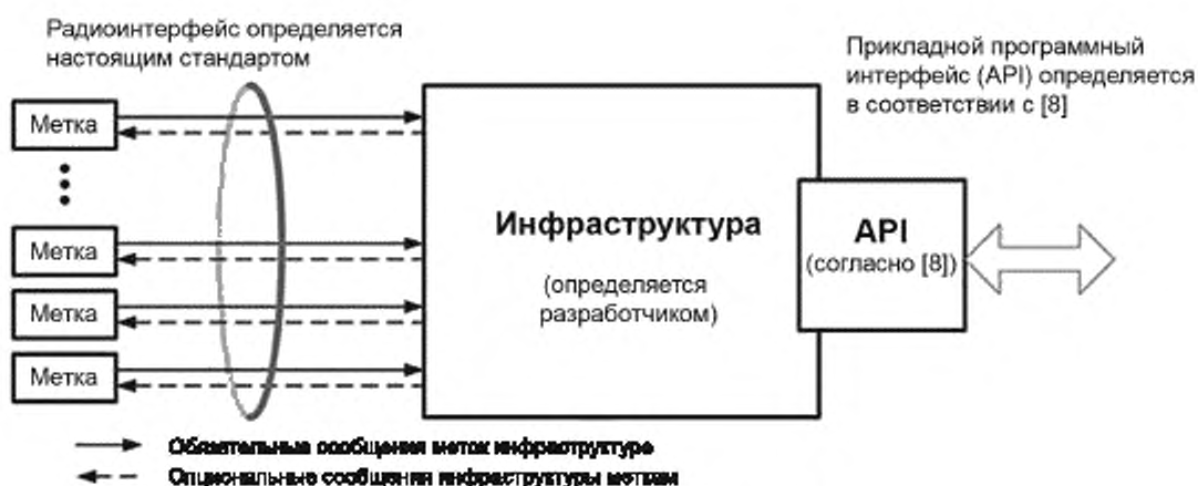
Рисунок 1 — Составные части системы RTLS
