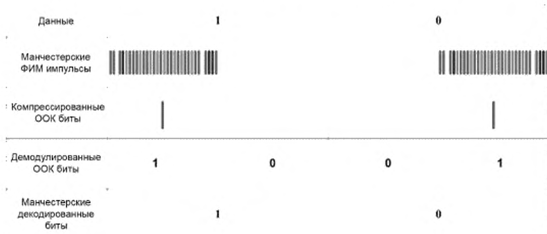
Рисунок А.2 — Преобразование Манчестерского кода двоичной фазоимпульсной модуляции (ФИМ) в ООК с использованием аналогового сжатия импульсов
