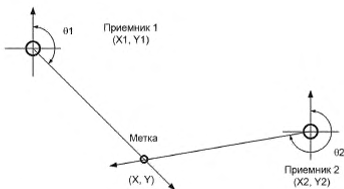
Рисунок А.5 — Определение местонахождения по угловым векторам
