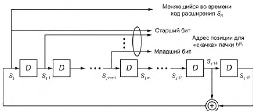
Рисунок 11 — Реализация скремблера в виде РСЛОС
