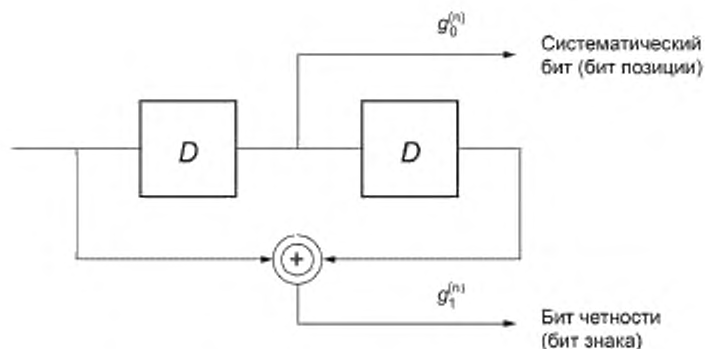
Рисунок 13 — Систематический сверточный кодер
