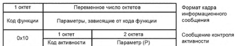
Рисунок 23 — Формат сообщения «контроль активности» (activity control)
