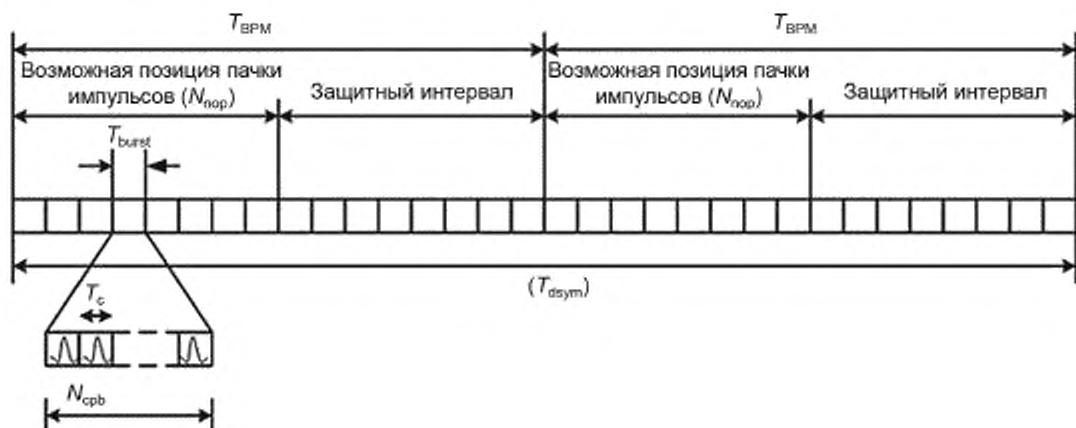
Рисунок 5 — Структура символа
