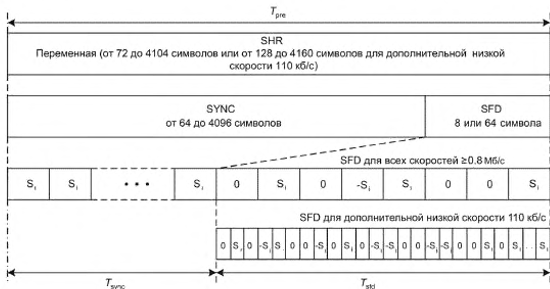
Рисунок 6 — Структура преамбулы SHR
