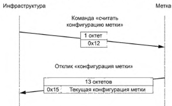
Рисунок 25 — Считывание конфигурации метки
