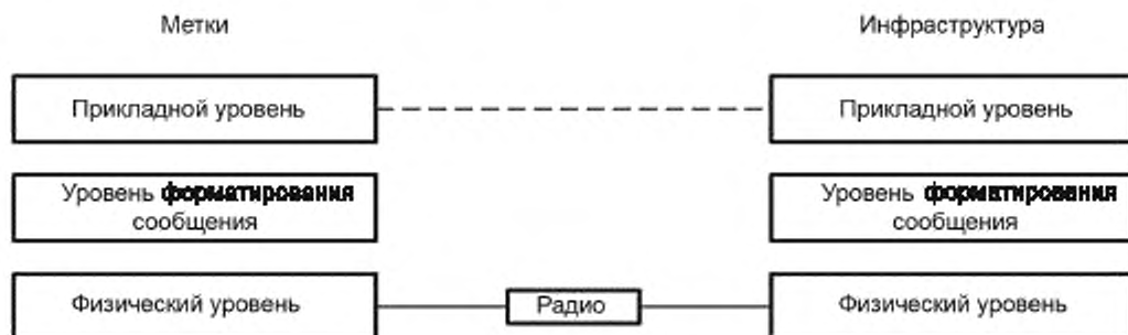
Рисунок 2 — Уровни радиоинтерфейса
