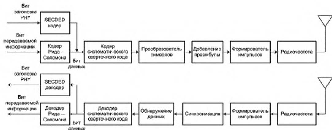
Рисунок 3 — Прохождение сигнала*
