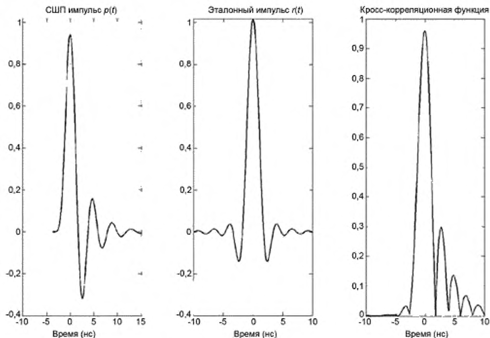
Рисунок 14 — Пример совместимого импульса
