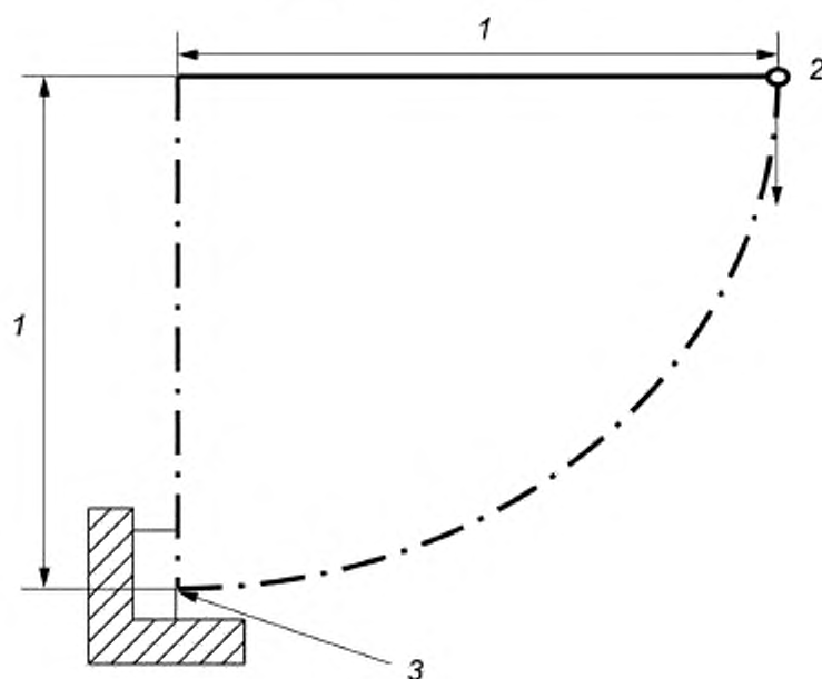
Схема движения маятника
