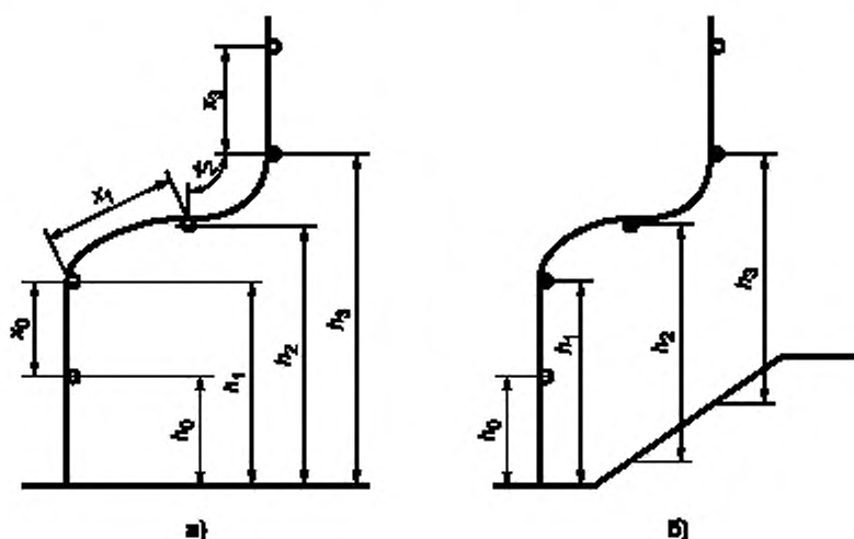
Рисунок 1 — Расположение точек страховки
