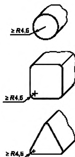
Рисунок 4 — Закругления деталей
