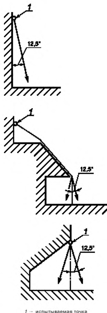
Рисунок Е.1 — Максимально допустимый угол направления приложения усилий
