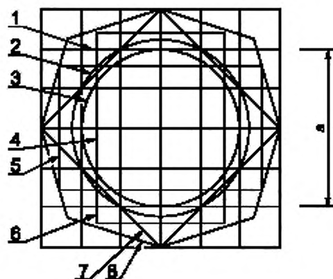
Рисунок 4.19 — Основная схема
