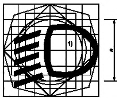
Рисунок 4.2 — Включение фар. Ближний свет
