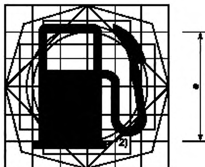
Рисунок 4.7 — Топливо
