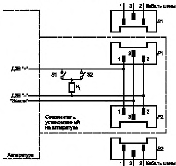
Рисунок Е.1 — Схема подключения аппаратуры к шине Д2В
