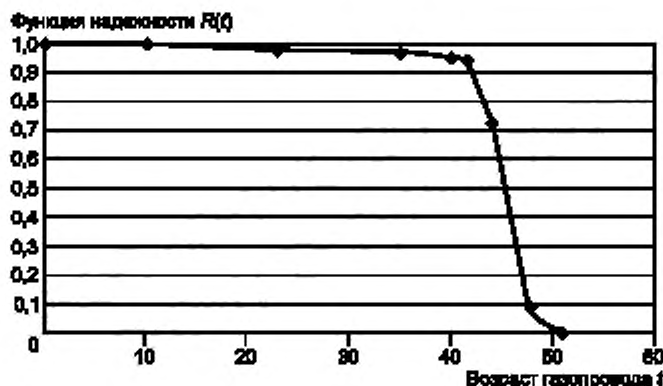
Рисунок Б.1 — График эмпирической функции надежности R(t)
