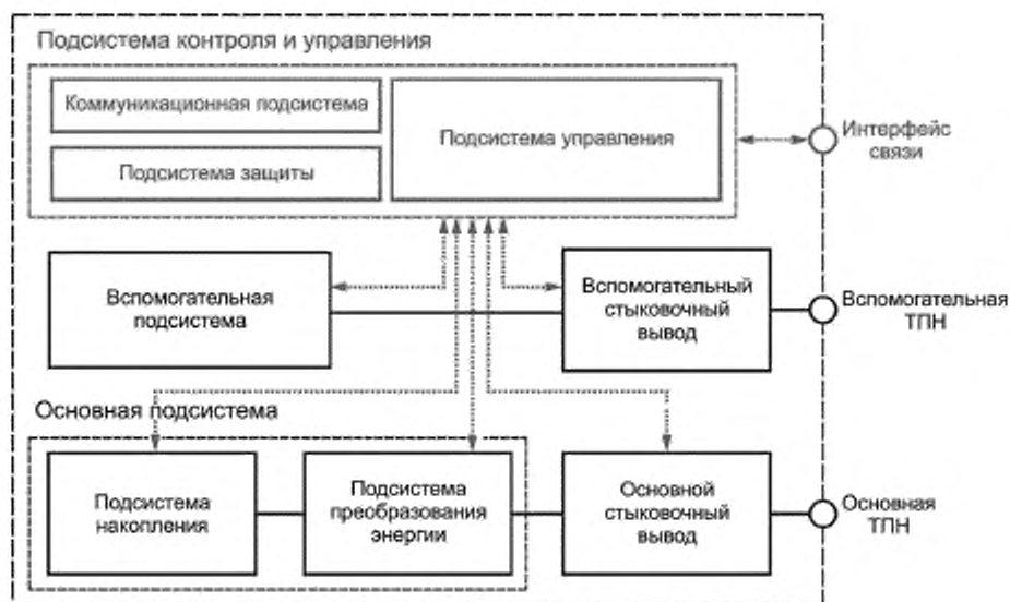
Рисунок 8 — Архитектура СНЭЭ в двух основных конфигурациях, лист 1
