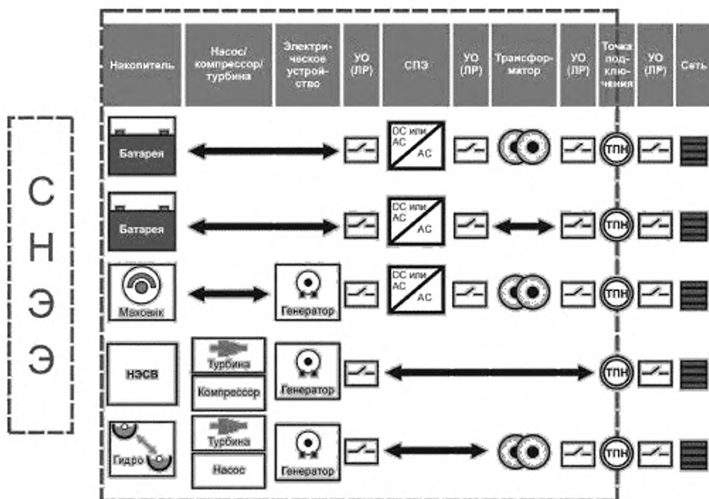
НЭСВ — накопитель энергии на сжатом воздухе; СПЭ — система преобразования энергии; УО — устройство отключения; ЛР — линейный разъединитель
