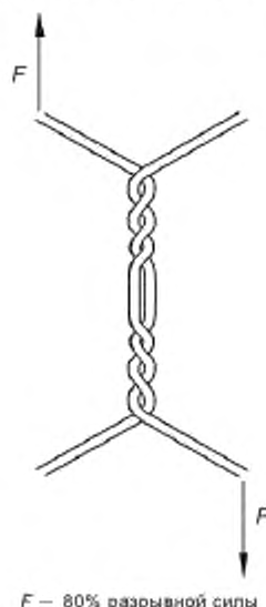
Рисунок 4 — Нагрузка на сетку для проверки прочности свивки
