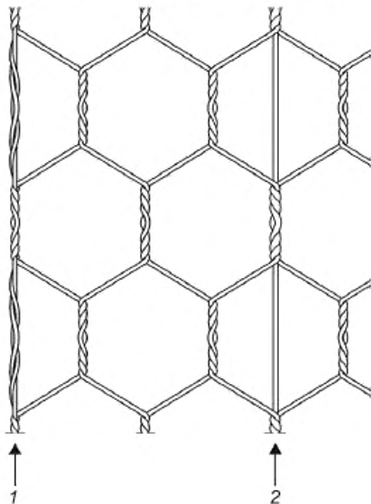
1 — бортовая проволока; 2 — проволочная растяжка
