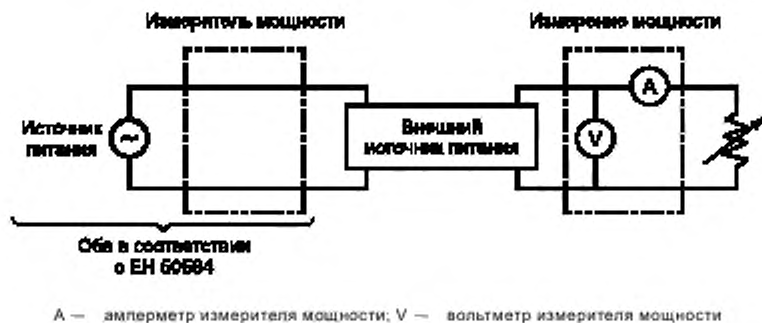
Рисунок 1 — Схема испытания
