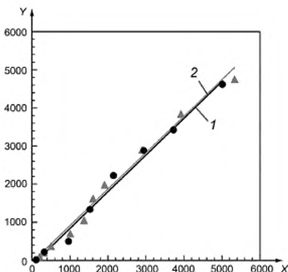
1 — диффузионная трубка; 2 — газовый баллон X — ГХ-МСД (толуоловый эквивалент, мкг/м 3 ); Y — ФИД (изобутиленовый эквивалент, мкг/м 3 )
