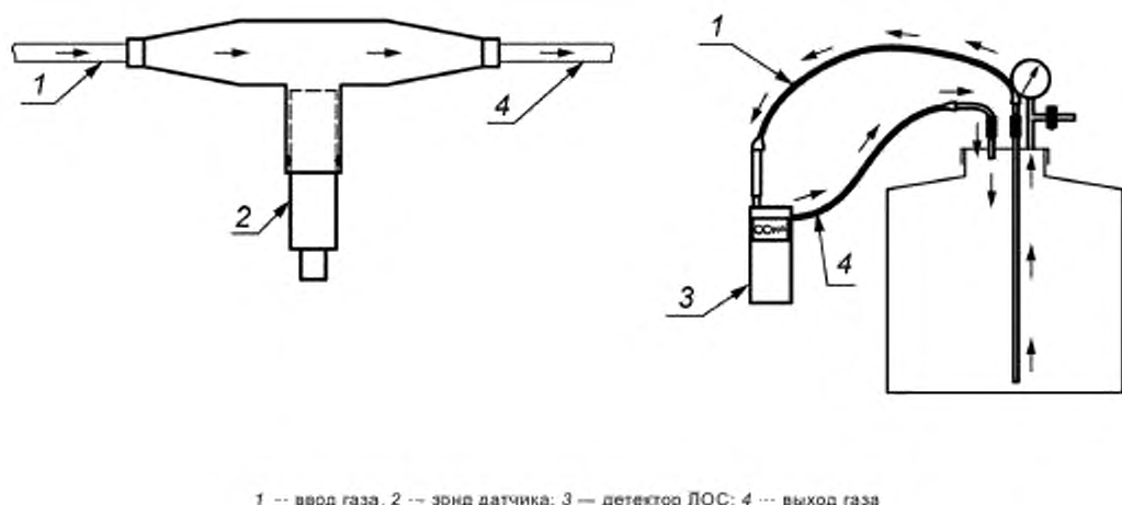
Рисунок В.1 — Маска (слева), испытательное оборудование камерного типа (справа)
