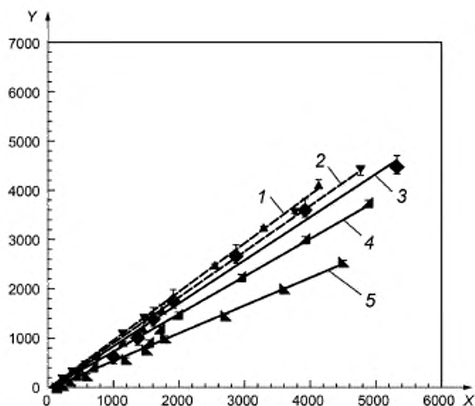
1 — шестикомпонентная смесь; 2 — искусственная газовая смесь; 3 — газ РМ; 4 — газ РВ; 5 — газ МВ X — ГХ-МСД (толуоловый эквивалент, \text{мкг}/\text{м}^3 ); Y — ФИД (изобутиленовый эквивалент, \text{мкг}/\text{м}^3 )
