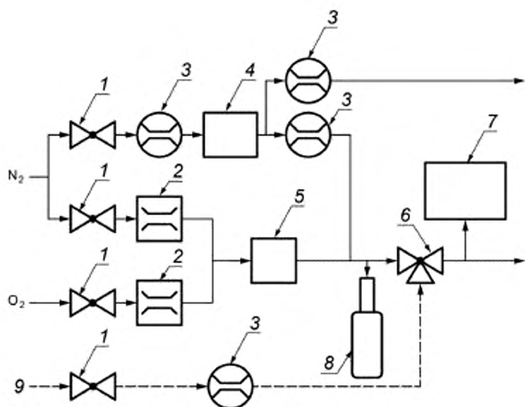
1 -- клапан, 2 -- регулятор массового потока, 3 -- расходомер с игольчатым клапаном; 4 -- газогенераторная система; 5 -- барботажное устройство, 6 -- трехходовой клапан, 7 -- ГХ.МСД, 8 -- портативный детектор ЛОС; 9 -- газовый баллон ЛОС
