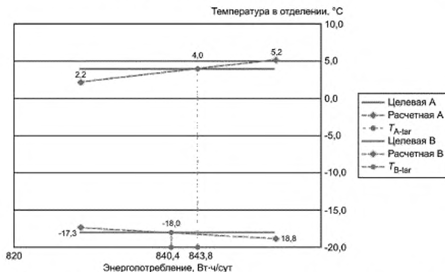
Рисунок I.4 — Пример интерполяции, когда в обеих точках испытаний оба отделения имеют температуру ниже целевой температуры (два допустимых результата)
