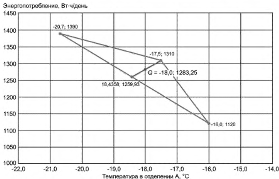
Рисунок I.9 — Пример триангуляции (температура и энергопотребление)
