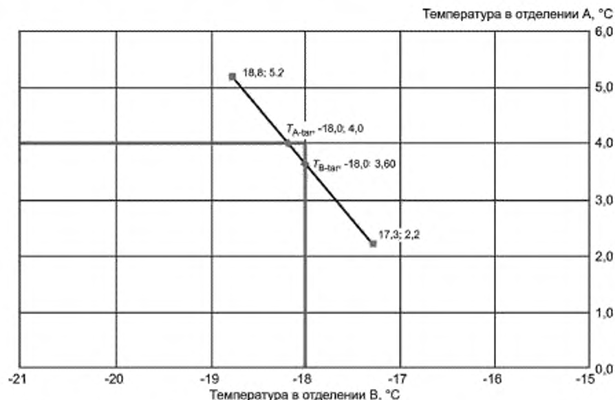
Рисунок I.3 — Пример интерполяции, когда в обеих точках испытаний оба отделения имеют температуру ниже целевой температуры (два допустимых результата)
