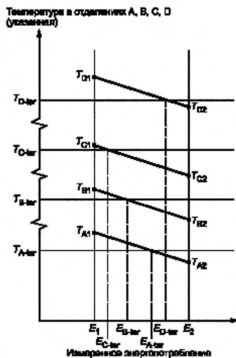
Рисунок E.1 — Интерполяция при изменении температур в нескольких отделениях (критическое значение для отделения D)
