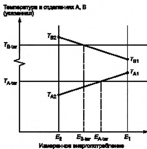
Рисунок E.2 — Интерполяция с корректными результатами в отделениях А и В
