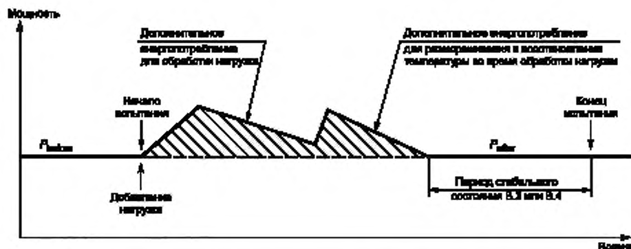
Рисунок G.5 — Пример, когда период размораживания и восстановления температуры происходит во время обработки загрузки
