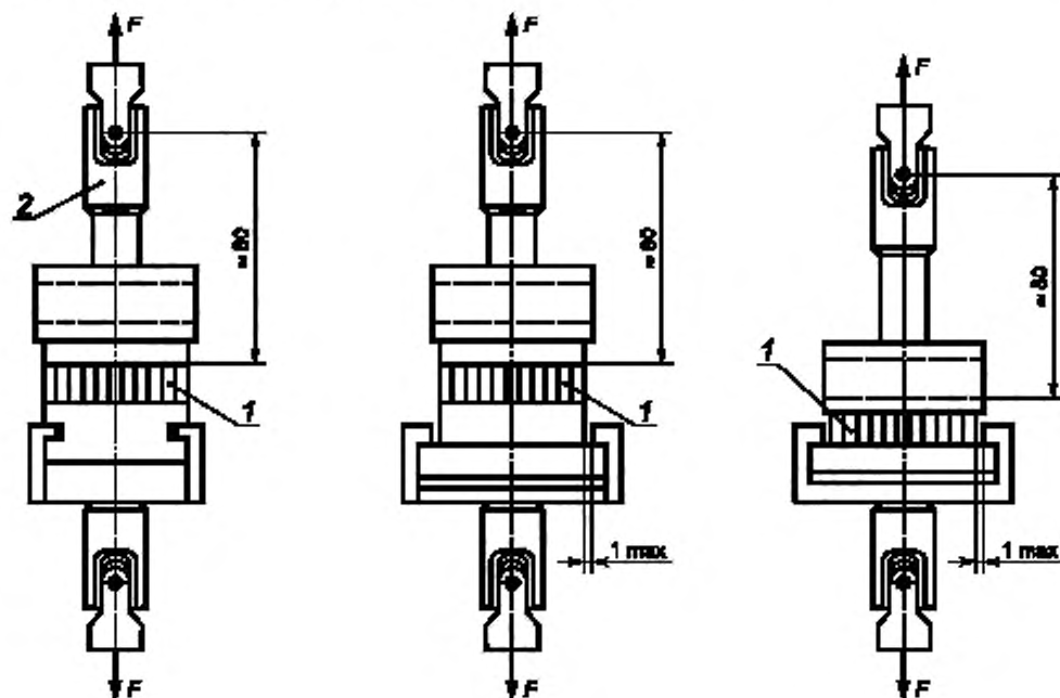
Рисунок 2 — Испытательное устройство
