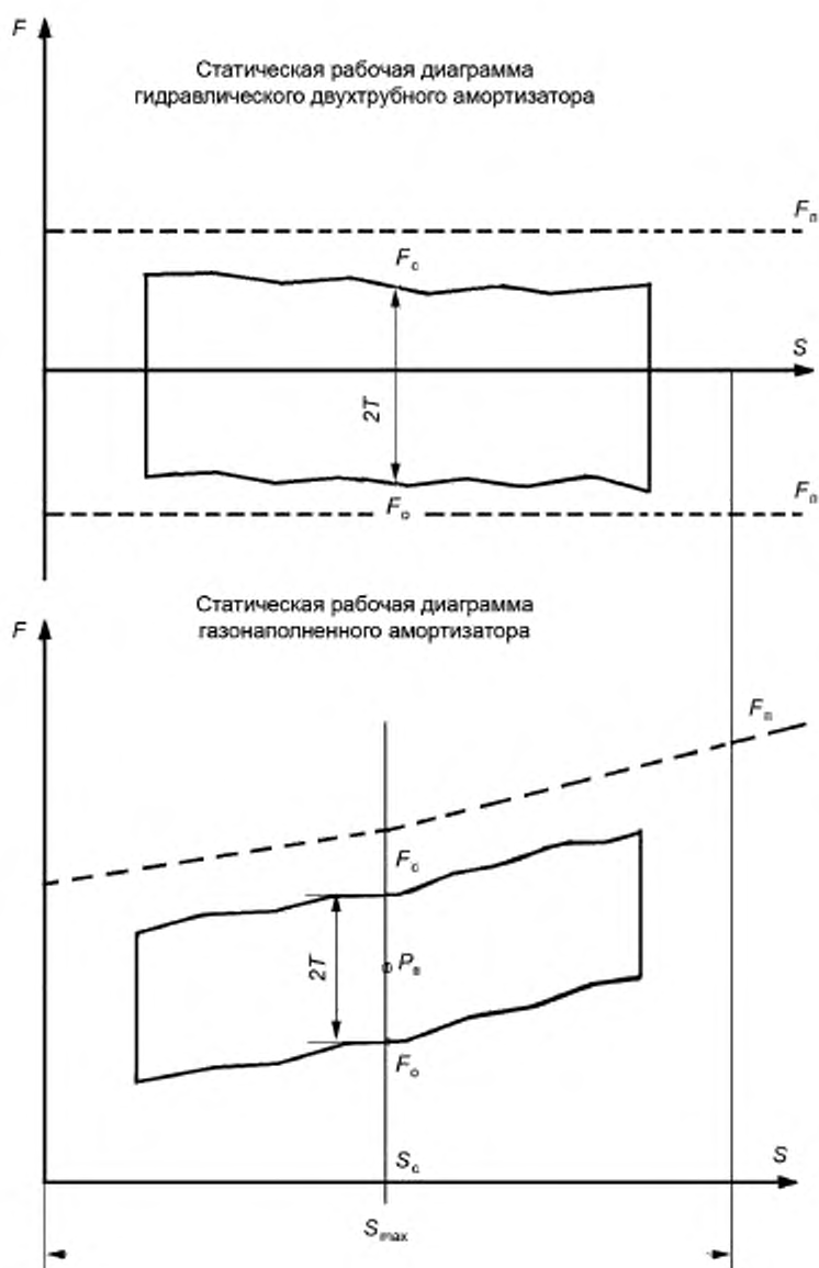
Рисунок 1 — Статические рабочие диаграммы амортизаторов
