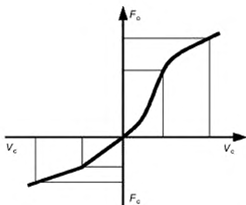
Рисунок 4 — Зависимость сопротивления амортизатора от скорости перемещения поршня
