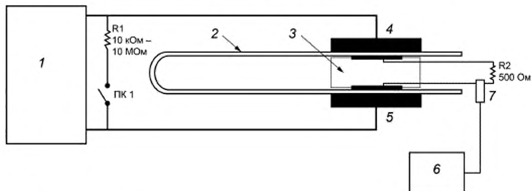
1 — ЭСР имитатор (обычно 100 пФ и 1500 Ом), 2 — испытуемый пакет, 3 — емкостный пробник; 4 — разрядный электрод; 5 — заземляющий электрод; 6 — осциллограф; 7 — токовый пробник
