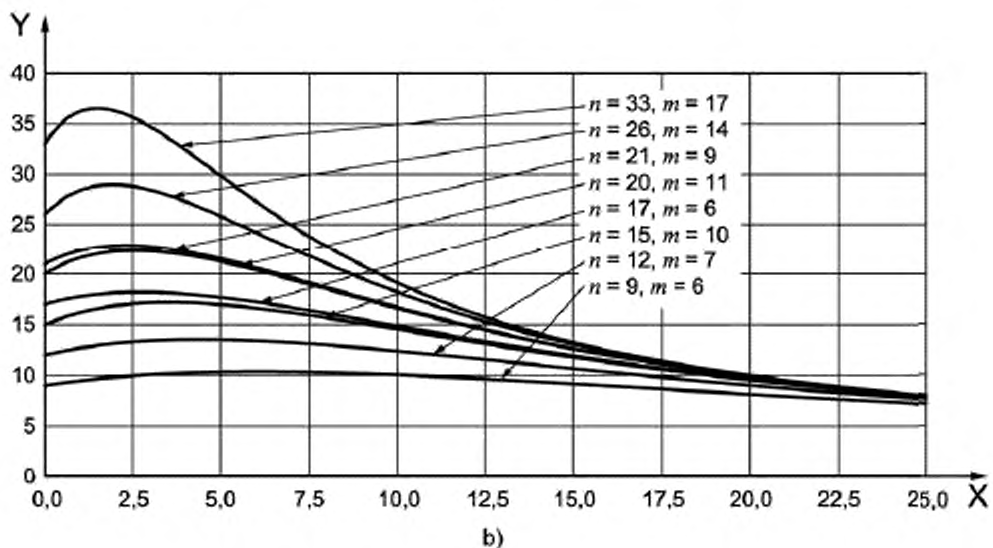
Рисунок 19 — Кривые среднего объема выборки для планов контроля доли несоответствующих единиц продукции, усеченный контроль с \alpha \leq 5\% и \beta \leq 5\%
