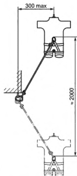
Рисунок 5 — Испытание на динамическую прочность
