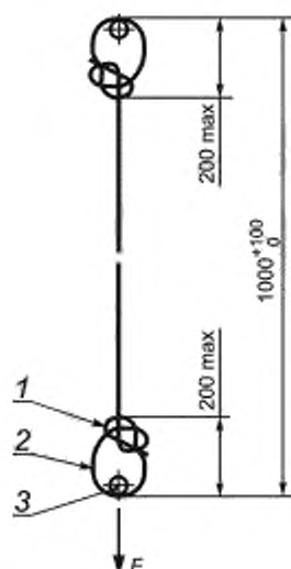
F — испытательный груз массой (100 + 1) кг или эквивалентная сила; 1 — узел булинь, 2 — петля заделки на конце; 3 — точка крепления
