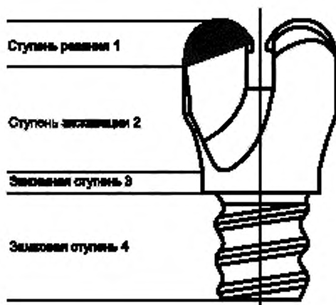
Рисунок 2 — Конструкция бурового резца
