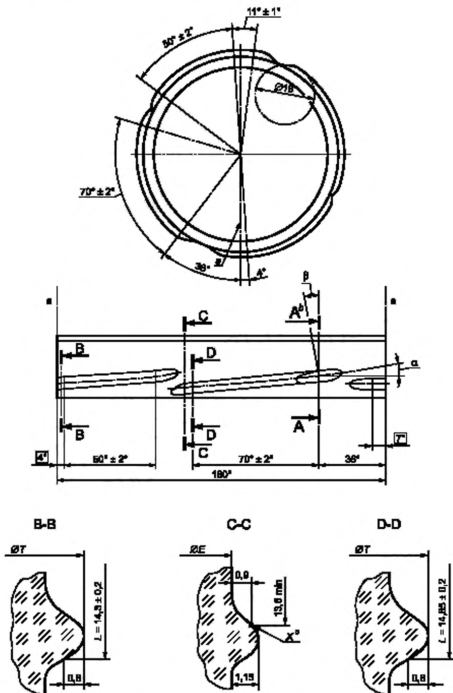
Рисунок 2 — Конструкция и увеличенные детали резьбы сечений В—В, С—С, D—D
