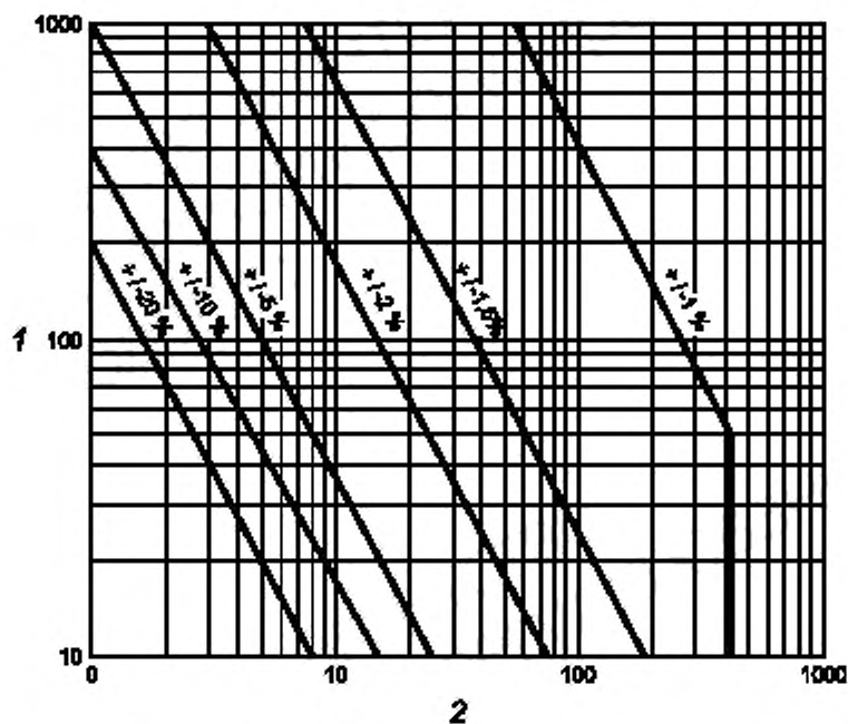
Рисунок D.1 — Рекомендованная остаточная пульсация давления
