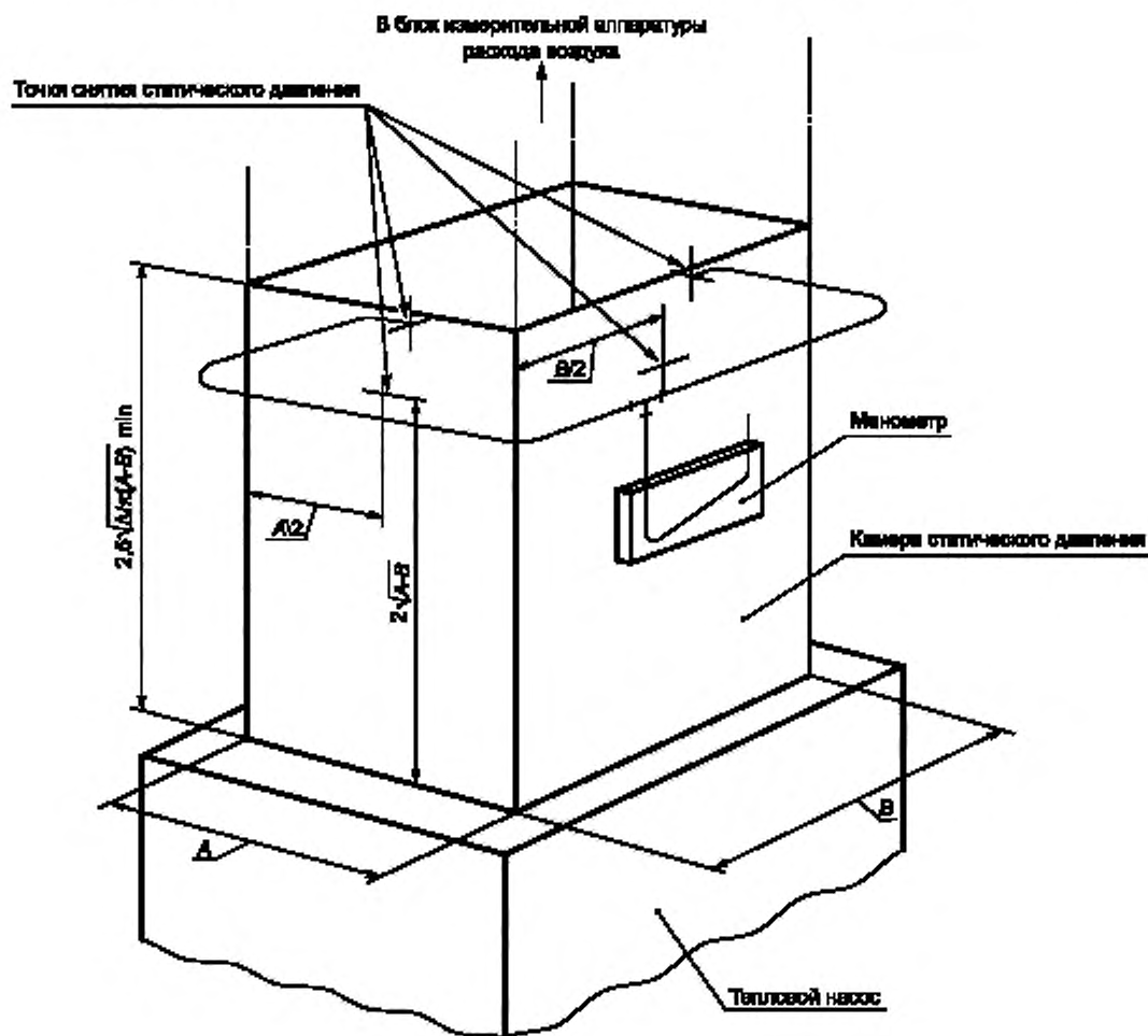
Рисунок F.7 — Измерение внешнего статического давления
