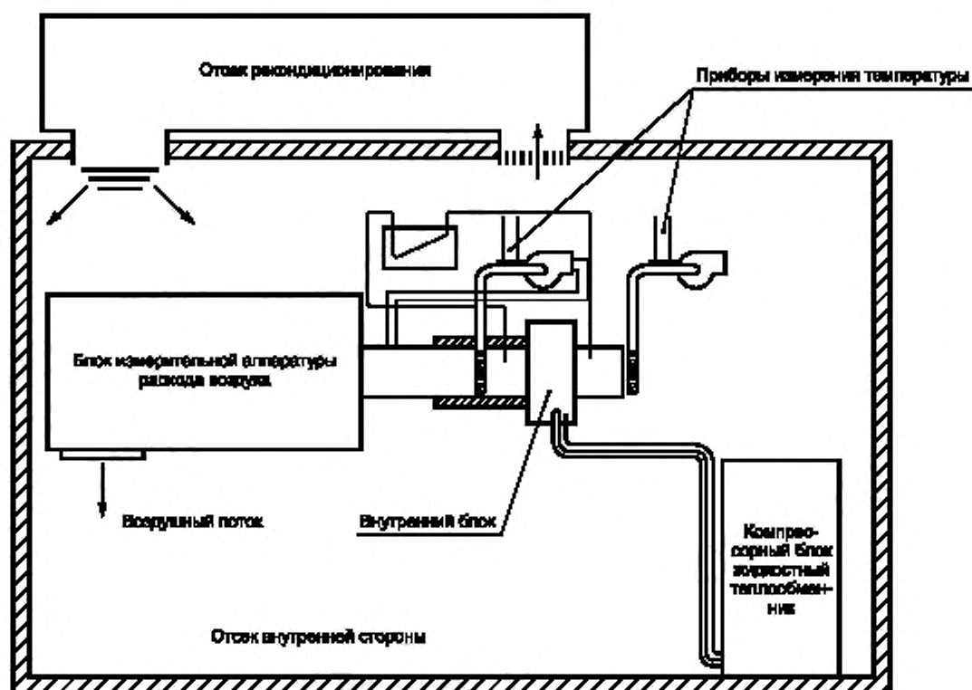
Рисунок F.1 — Компоновка оборудования испытательной камеры для проведения испытаний методом туннеля
