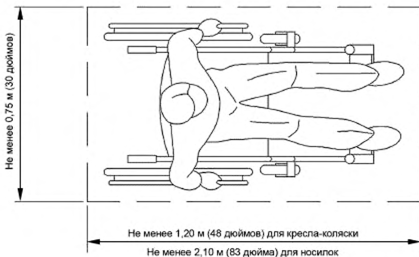
Рисунок А.1 — Чистая площадь пола
