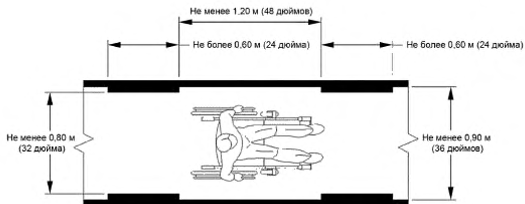
Рисунок А.2 — Свободная ширина прохода
