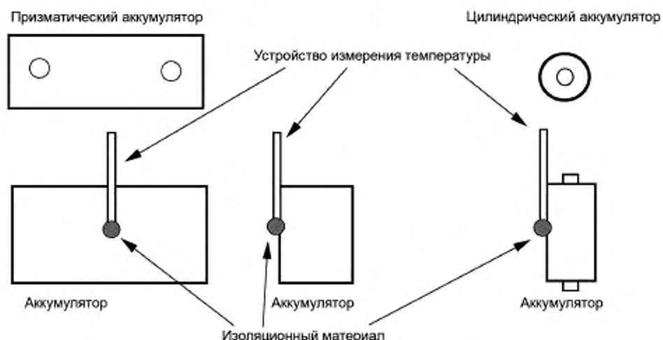
Рисунок А.1 — Пример измерения температуры аккумулятора
