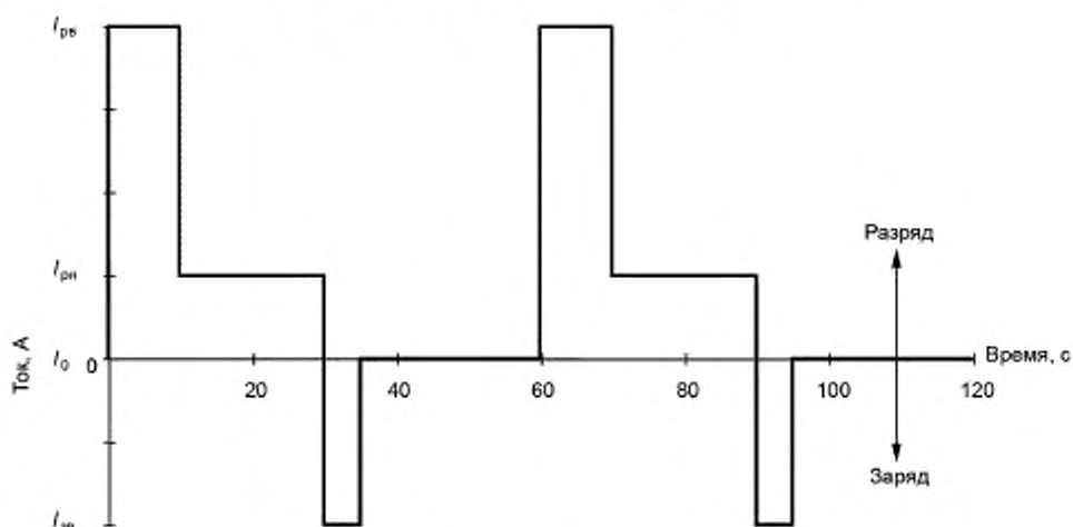
Рисунок 2 — Профиль испытания с рекуперацией
