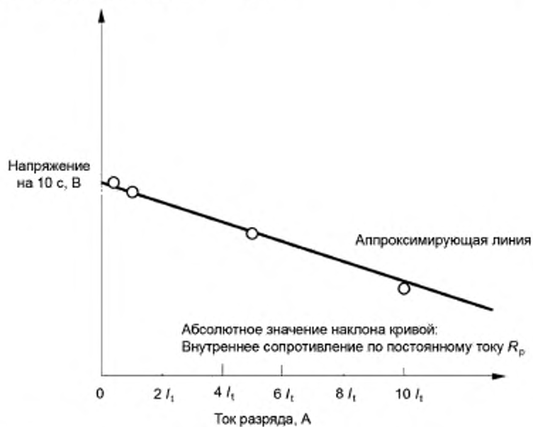
Рисунок А.6 — Метод получения значения внутреннего сопротивления по постоянному току при разряде
