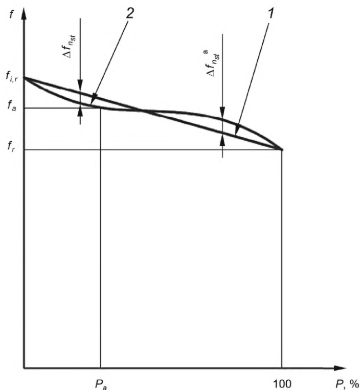
P — мощность; f — частота; 1 — линейная кривая характеристики быстрогодействия мощности; 2 — кривая частотно-энергетической характеристики
