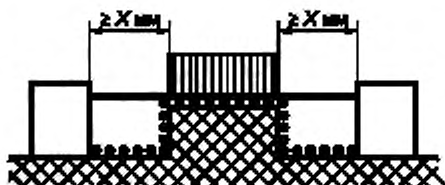
Рисунок AA.5 — Нескрепленный стык с узким желобком
