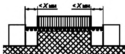
Рисунок AA.4 — Ребро
