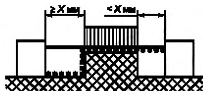
Рисунок AA.6 — Нескрепленный стык с широким желобком
