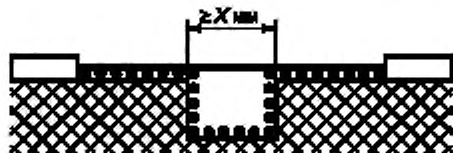
Рисунок АА.1 — Узкий желобок
