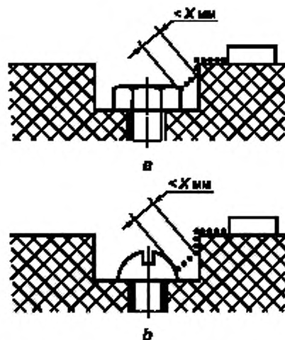
Рисунок АА.9 — Узкий паз
