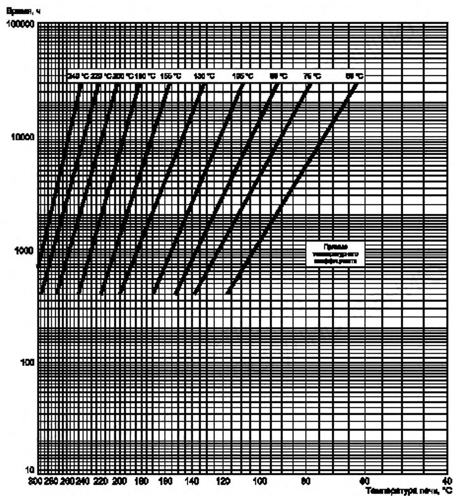
Рисунок E.1 — Длительность испытания в зависимости от температуры печи для предлагаемого температурного коэффициента
