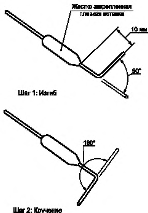
Рисунок 1 — Изгибающая/скручивающая сила
