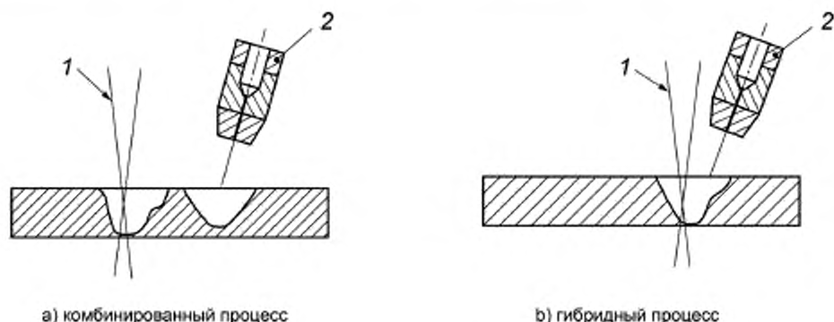
Рисунок 1 — Комбинация сварочных процессов
