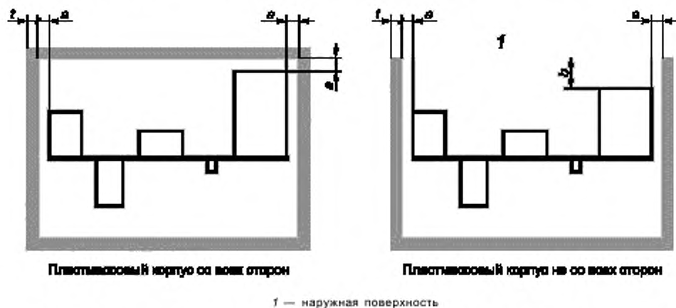
Рисунок 3 — Расстояния между стенкой или наружной поверхностью компаунда и элементами или проводниками
