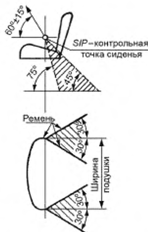
Рисунок Б.1 — Места крепления ремней безопасности
